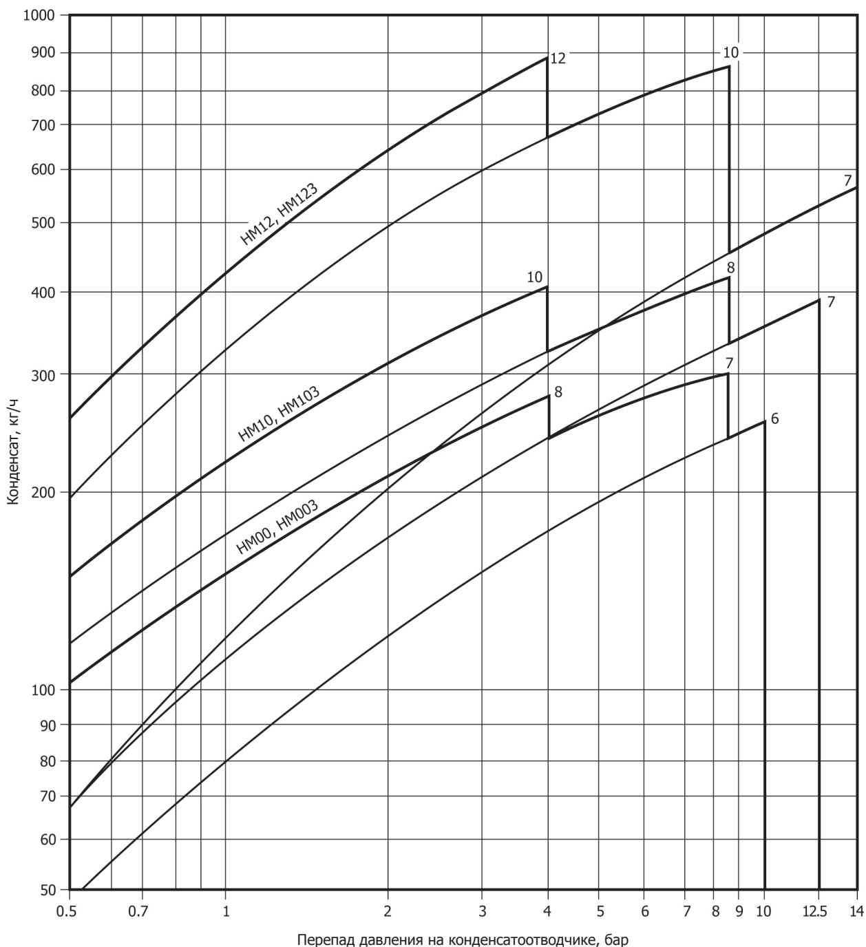
Пропускная способность конденсатоотводчиков серии НМ
