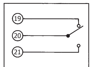
Настраиваемые концевые выключатели
