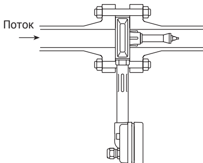
Рис. 8 Ограничение по давлению до 32 бари
