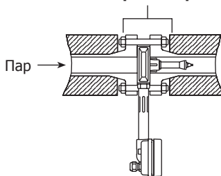
Рис. 5 Теплоизоляция паропровода
