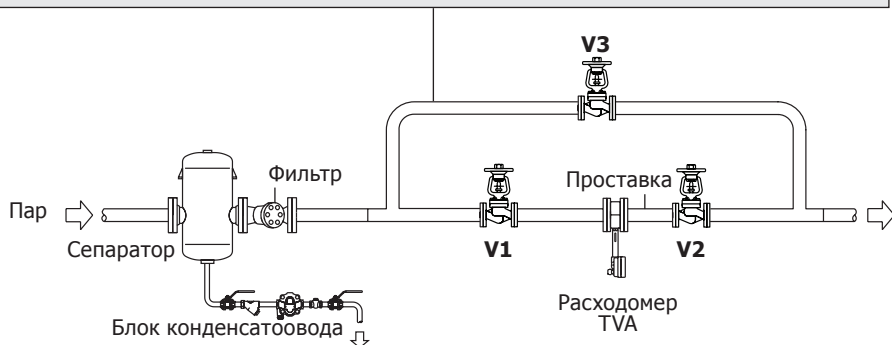
Рис. 4 Типовая схема монтажа
