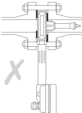
Рис. 16 Неправильно установленные прокладки
