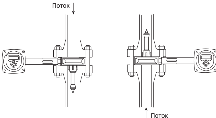
Рис. 6 При установке на вертикальном трубопроводе ограничение по давлению пара: 7 бари
