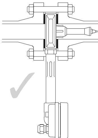
Рис. 15 Правильно установленные прокладки
