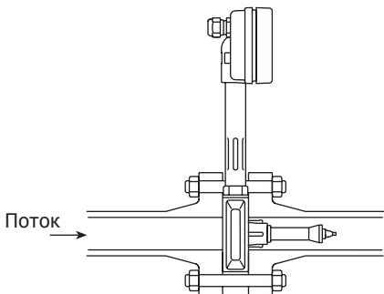
Рис. 7 При установке на горизонтальном трубопроводе при блоке электроники сверху ограничение по давлению пара 7 бари
