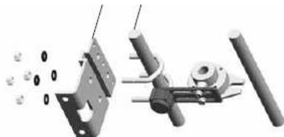
Rys. 9 Montaż płytki na siłowniku kolumnowym
