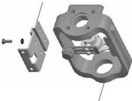
Rys. 10 Montaż płytki na siłowniku jarzmowym
