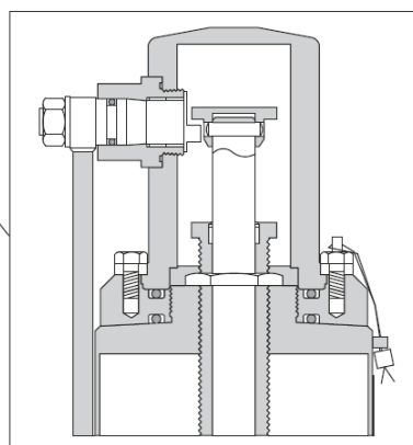
Gasdichte hefboom DN40 (1.1/2") en groter
