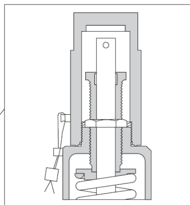
Gasdichte kap Alle maten
