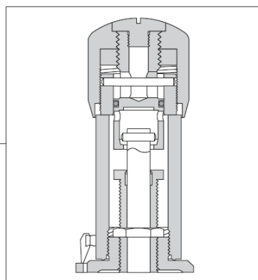
Gasdichte hefboom DN25 (1")
