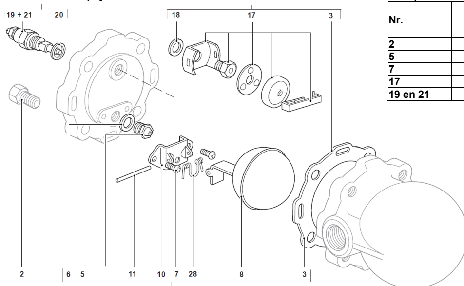
Set mechanisme met vlotter Opmerking : Nr. 28 alleen voor 1"
