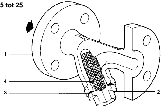
DN 32 tot 50
