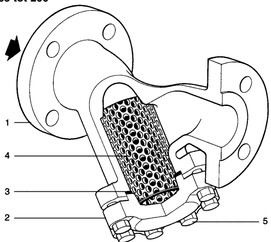
DN 65 tot 200
