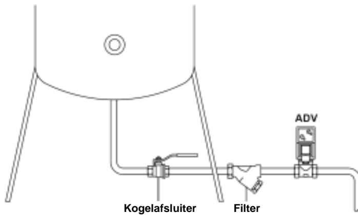
Fig.1 Spuien van een buffer of grote filter
