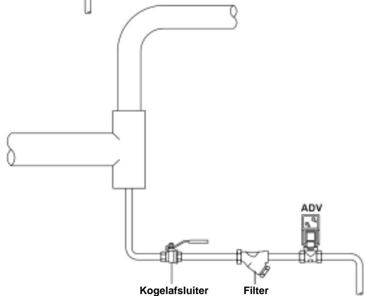
Fig.2 Leidingsontwatering persluchtnet
