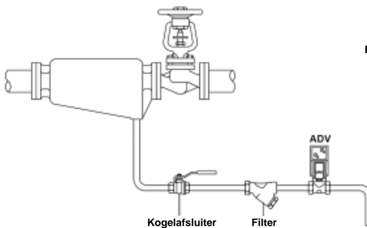
Fig.3 Ontwatering waterafscheider persluchtnet
