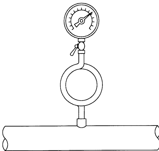
Horizontale leiding (moet voldoende ruimte)
