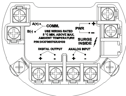
Fig. 29 VLM30E-klemmen
