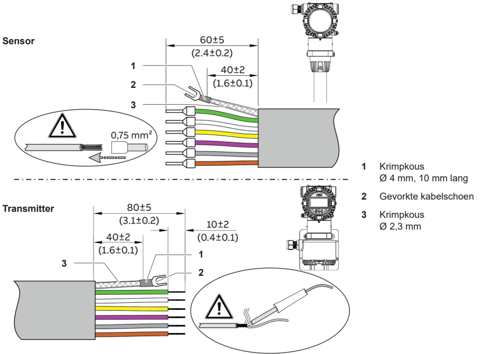
Fig. 31 Signaalkabel, afmetingen in mm (")
