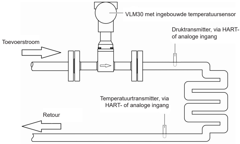
Fig. 38 Energiemeting
