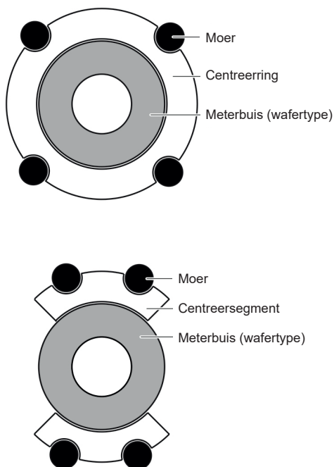
Fig. 15 Centrereren van de uitvoering van het wafertype met de ring of het segment
