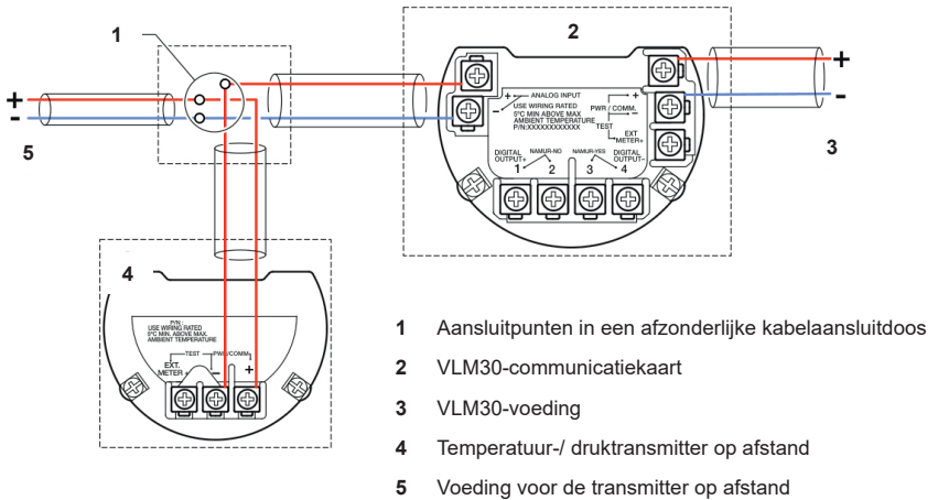
Fig. 25 Aansluiting van transmitters op een analoge ingang (voorbeeld)
