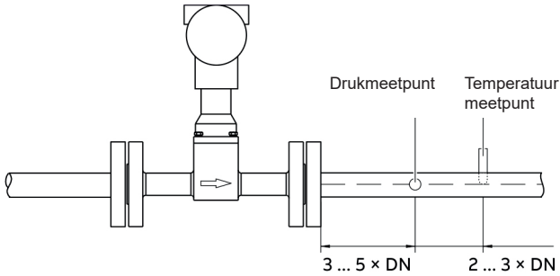
Fig. 8 Opstelling van de temperatuur- en drukmeetpunten
