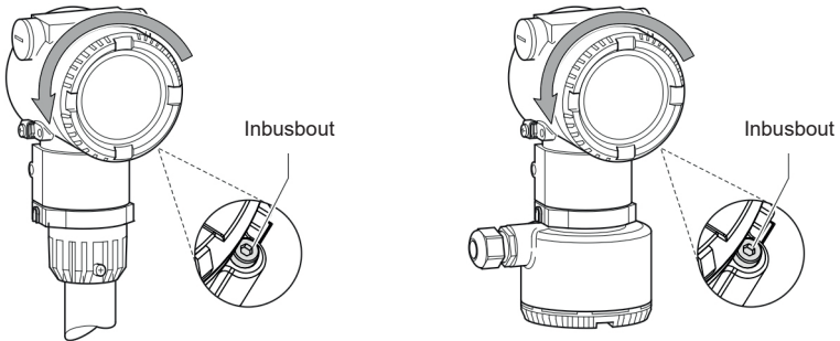
Fig. 18 Dekselvergrendeling (voorbeeld)
