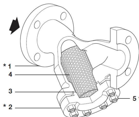
Y-Filter (met deksel met bouten)
