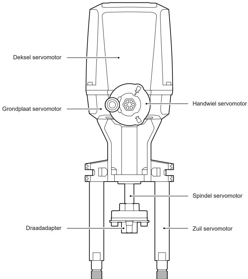
Fig. 1 AEL8 Algemene opstelling
