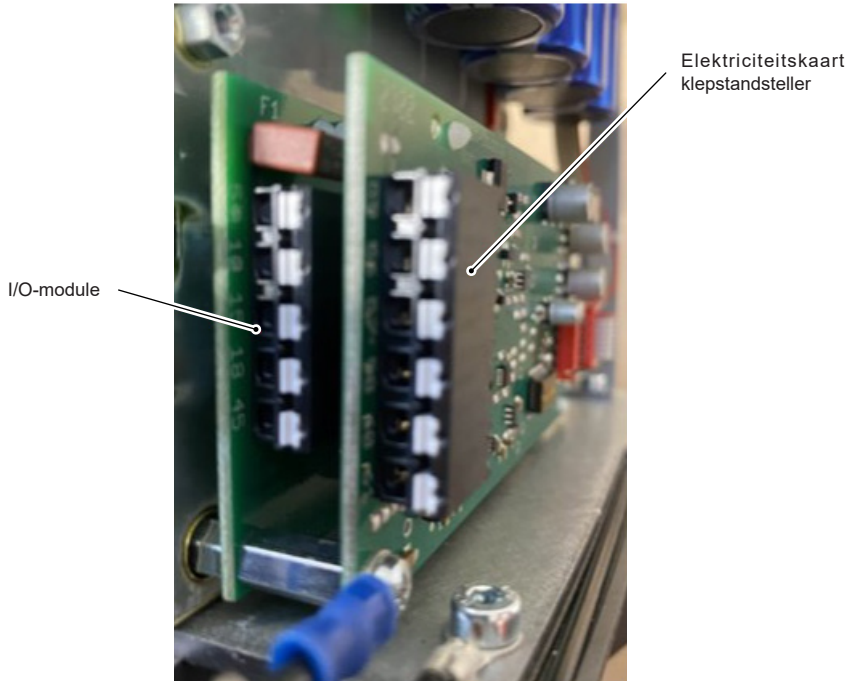
Fig. 5 PEL-richting
