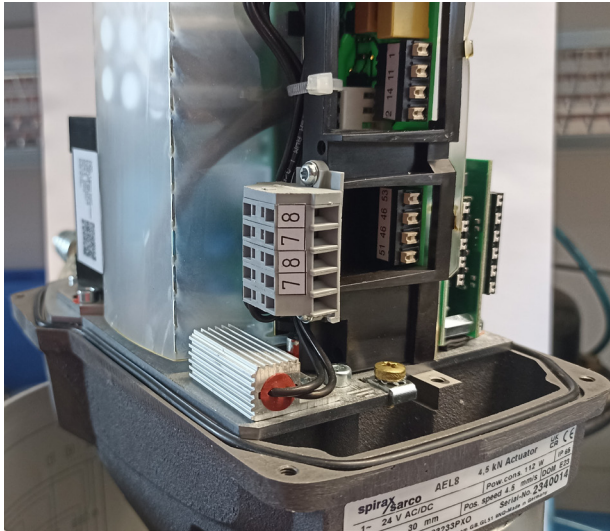
Fig. 7 Oriëntatie I/O-heater
