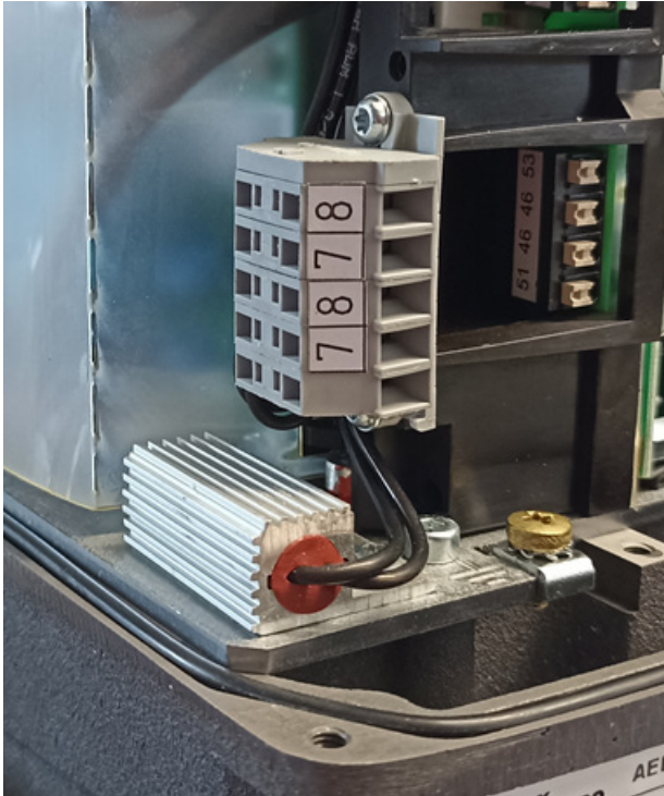
Fig. 6 I/O-module oriëntatie
