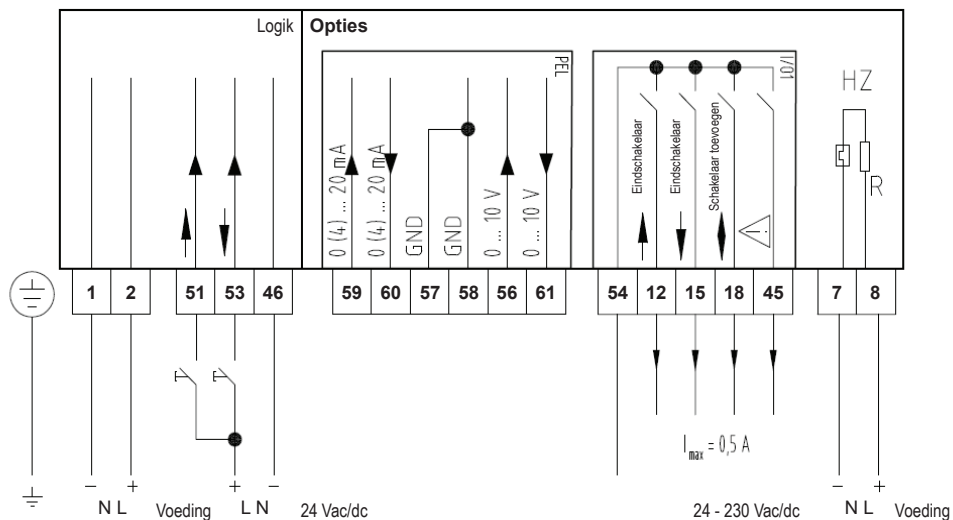
Fig 4. AEL8 aansluitschema 100-240 Vac
