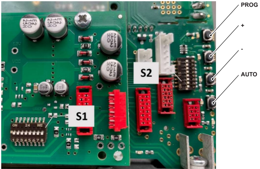
Fig. 7 Elektronische kaart klepstandsteller
