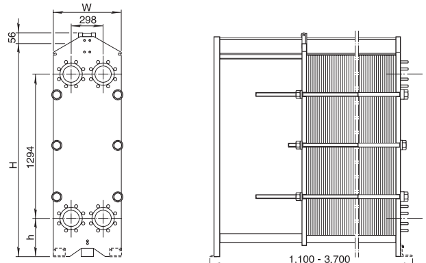
T15B-FG 치수
