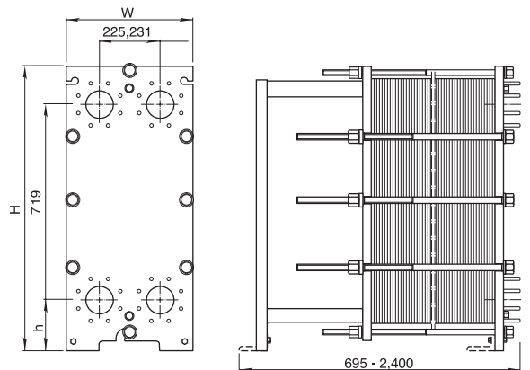
T10B-FG 치수
