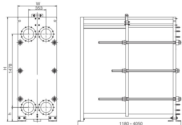
M20-MFG 치수
