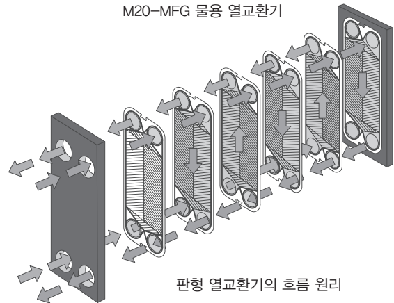
M20-MFG 물용 열교환기
