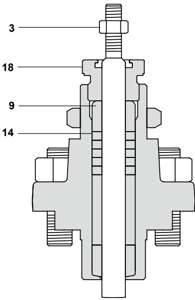
KE 밸브 그라파이트 패킹
