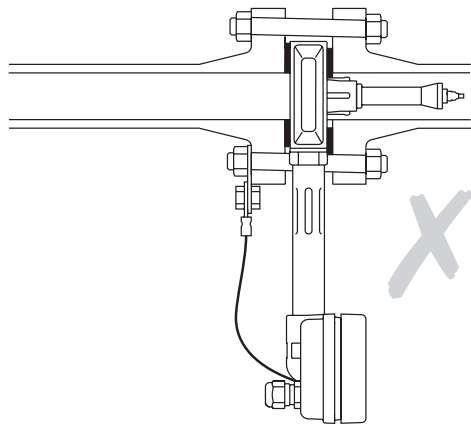
그림 18. 잘못 설치된 가스켓과 오정렬 배관
