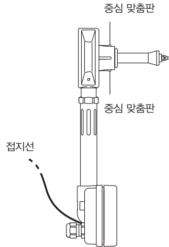
그림 15. 중심 맞춤판
