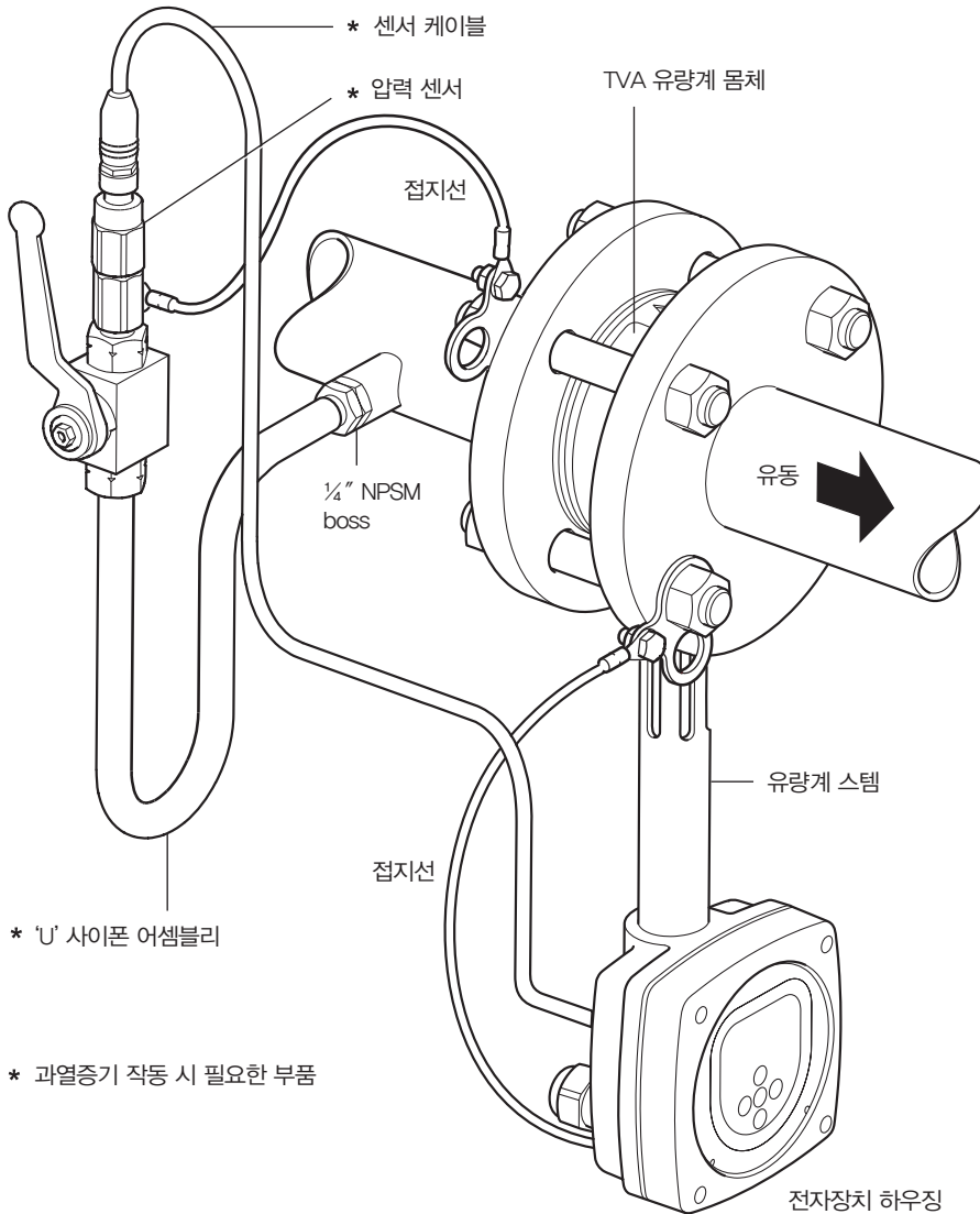
그림 19. TVA 유량계
