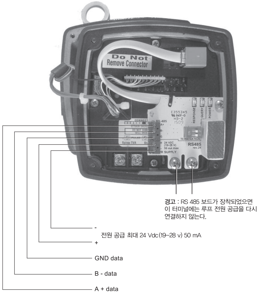
그림 21. TFA EIA 485(RS 485) 통신 배선도
