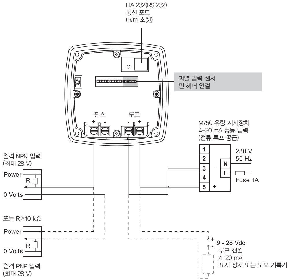
그림 20. EIA 232(RS232) 통신이 있는 TVA 4~20 mA 배선도
