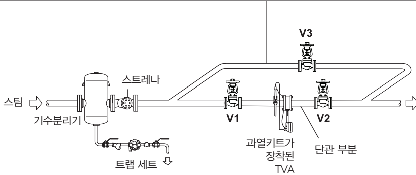
그림 5. 일반적 설치
