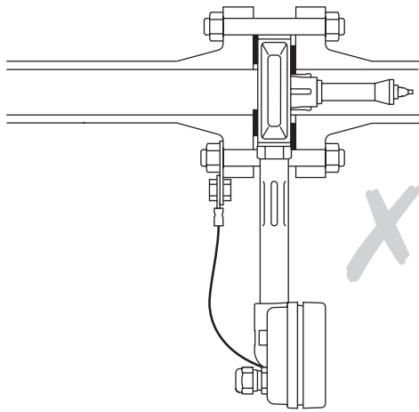
그림 17. 잘못 설치된 가스켓
