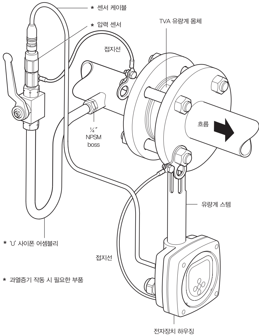
그림 1. TVA 유량계
