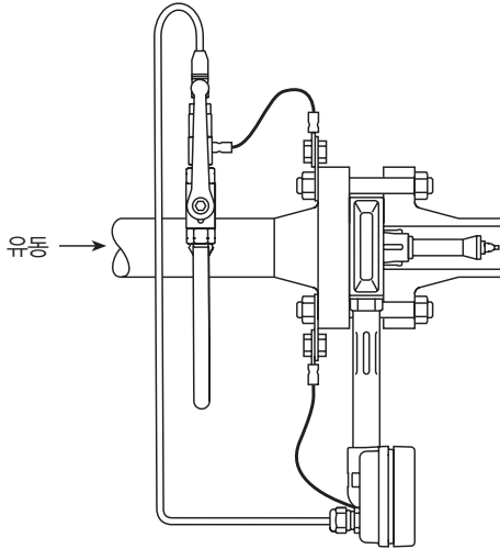
그림 9. 32 bar g까지의 포화증기 어플리케이션, 23 bar g까지의 과열증기 어플리케이션의 수평 유동
