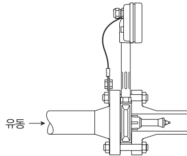
그림 8. 포화증기 어플리케이션의 7 bar g로 제한된 수평 유동
