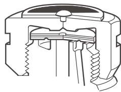
그림 2. TD32FLC, TD32FALC의 캡에는 홈이 있다.
