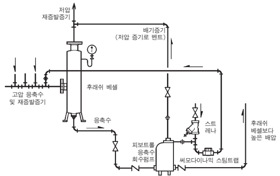
그림 10. 대기압 이상 또는 이하에서 재증발증기 회수
