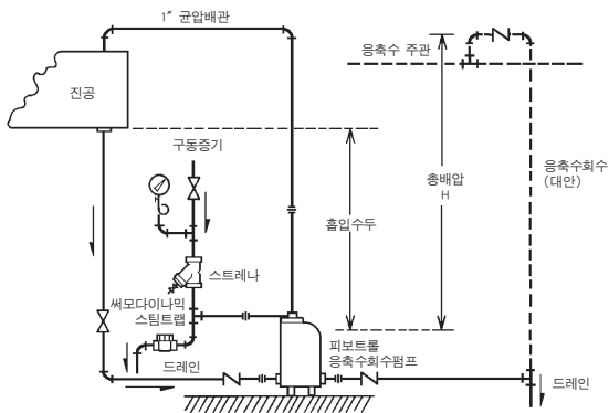
그림 11. 진공 공간에서 응축수회수
