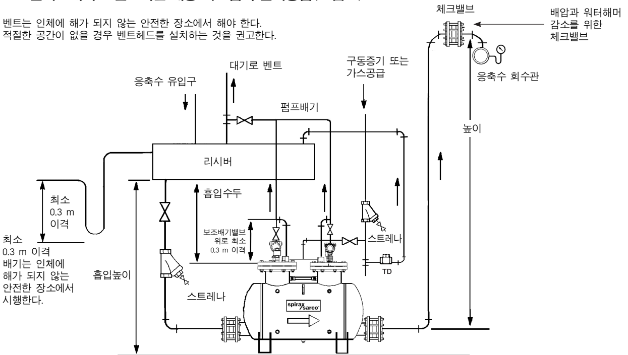
그림 2. 벤트 펌프 시스템
