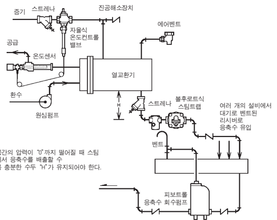
그림 12. 소형 열교환기에서 응축수회수
