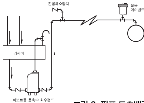
그림 8. 펌프 토출배관이 긴 경우
