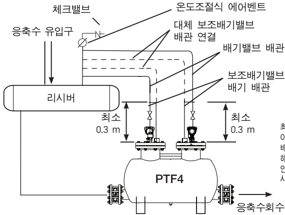
폐쇄 시스템에서의 PTF4 배기와 보조배기밸브 배관 연결
