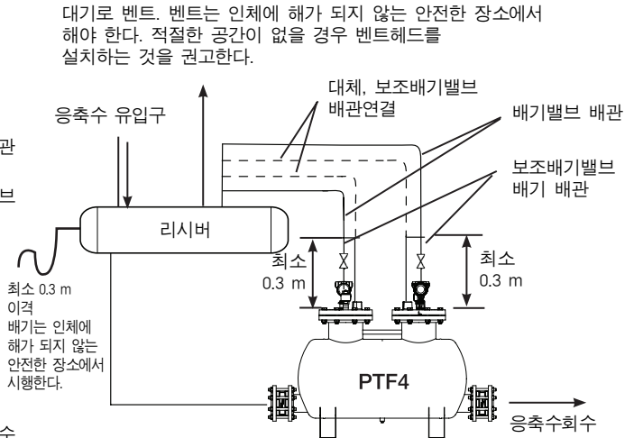
개방(벤트) 시스템에서의 PTF4 배기와 보조배기밸브 배관 연결
