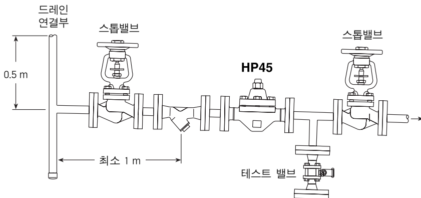
그림 3. 추천 설치방법(주 : 배관은 흐름방향으로 경사가 져야 한다.)
