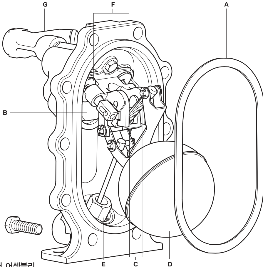
그림 12. 커버 어셈블리
