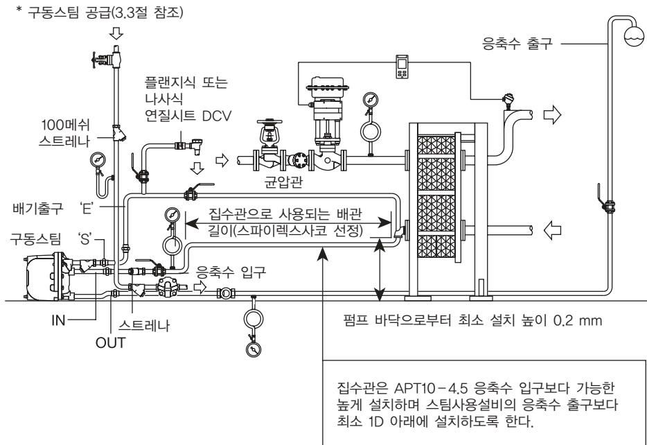
그림 4. 구동스팀 공급 및 배기관 연결도
