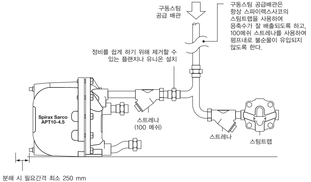
그림 4. 구동스팀 공급 및 배기관 연결도
