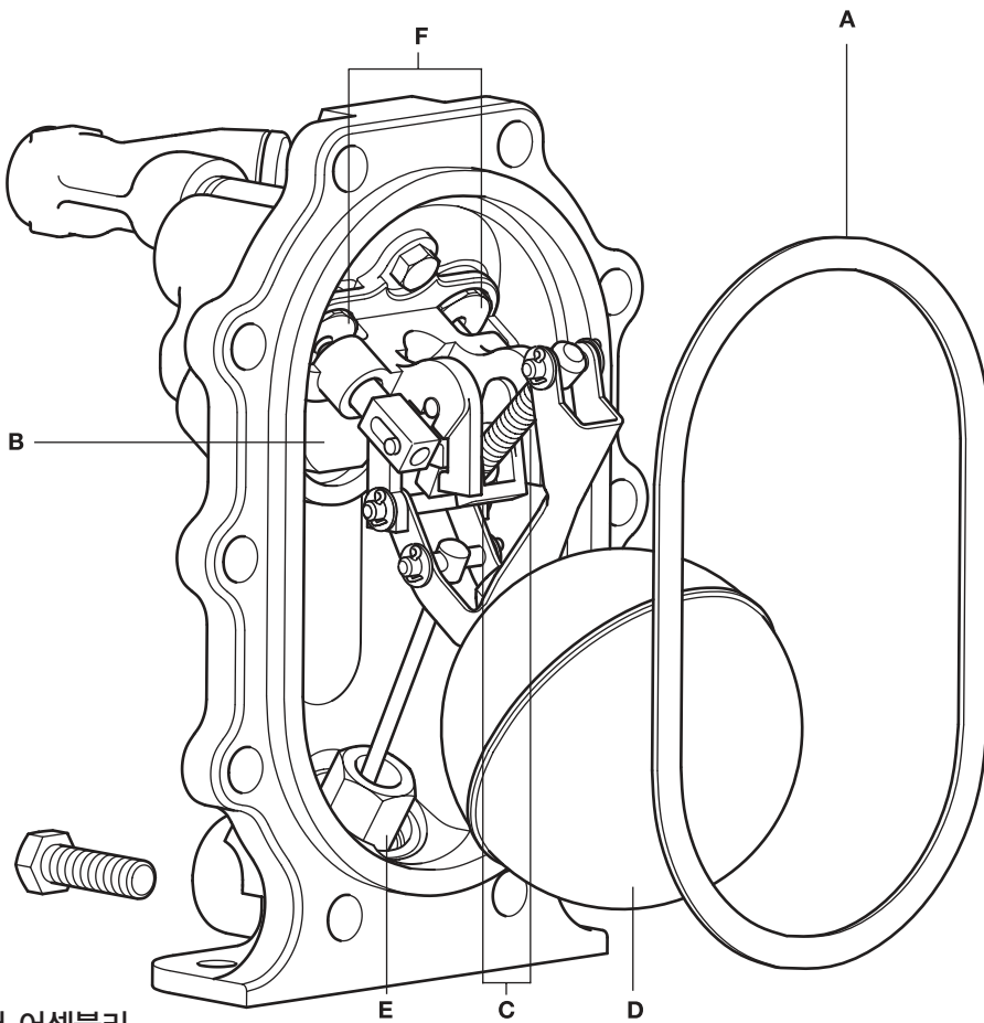
그림 13. 커버 어셈블리
