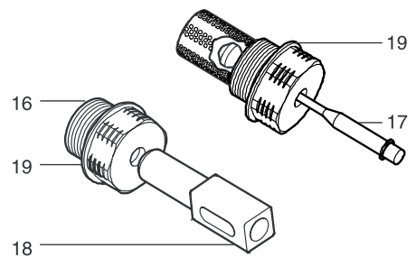
F 스팀공급/배기밸브 및 시트
