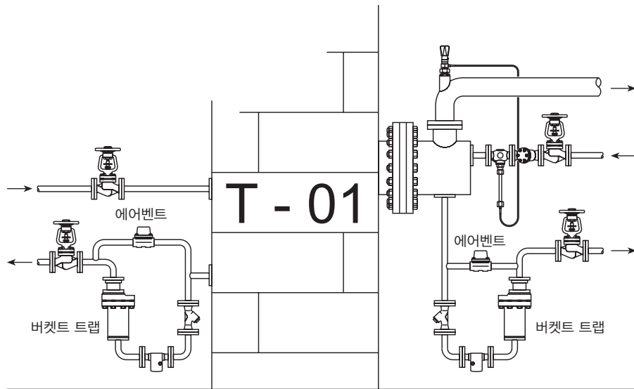
그림 3. 일반적인 설치방법-오일 저장 탱크
