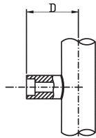
Codice S... Stub End Da saldare a tasca
