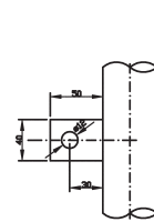
Staffa di supporto (raccomandata per A > 3000)
