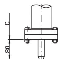
B... Giunto a saldare di testa
