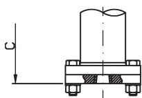
Codice F... / H... Attacco filettato femmina
