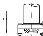
S... Attacco a saldare a tasca
