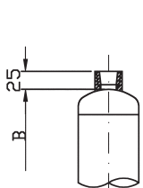
Codice F... / H... Attacco filettato femmina
