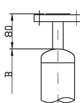
Codice U... / A... Attacco Flangiato
