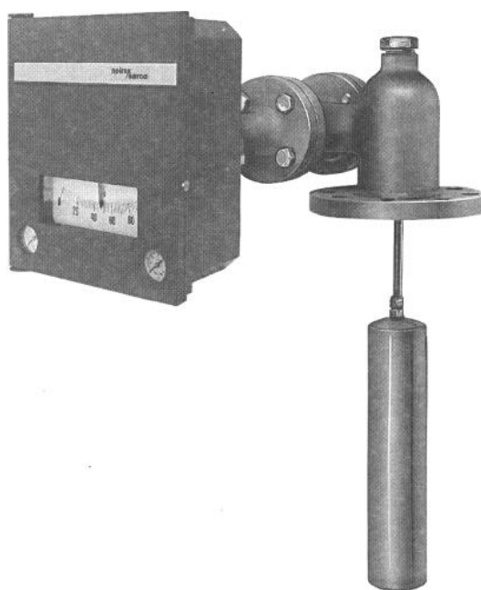
Fig. 3 - Strumento di livello per montaggio di testa interno
