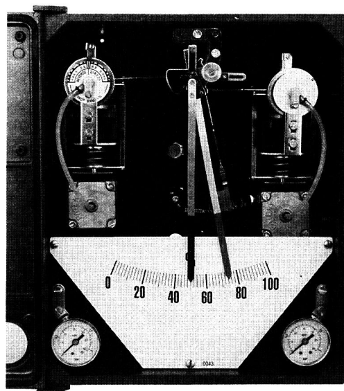
Fig. 7 - Vista interna di uno strumento trasmettitore regolatore
