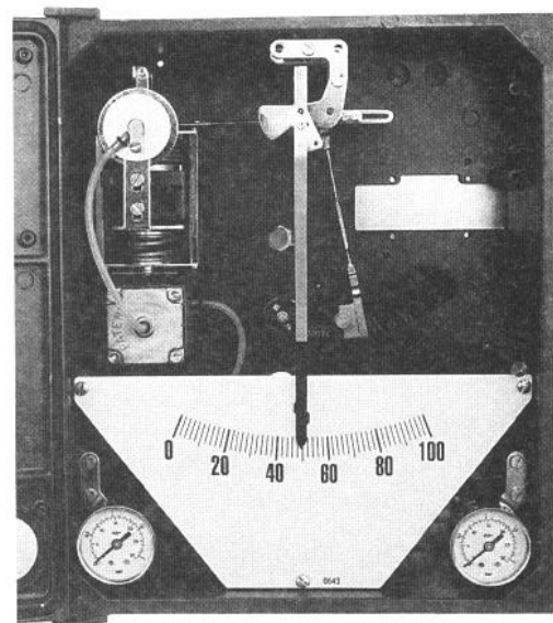
Fig. 5 - Vista interna di uno strumento trasmettitore
