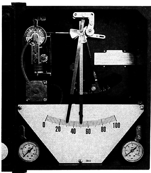
Fig. 6 - Vista interna di uno strumento regolatore
