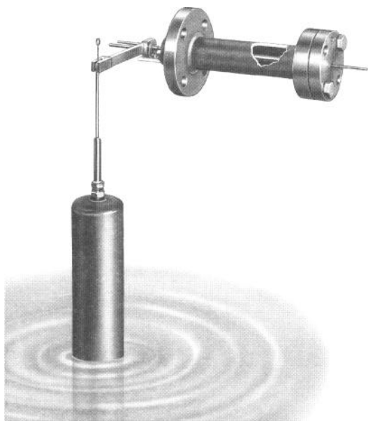
Fig. 4 - Gruppo dislocatore - tubo di torsione
