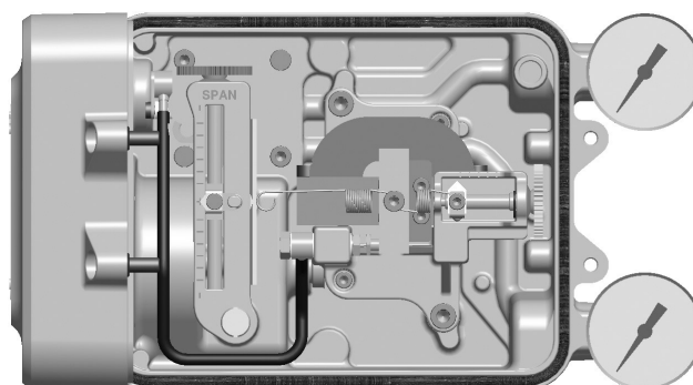
EP500 con pannello frontale aperto per visualizzare l'interno
