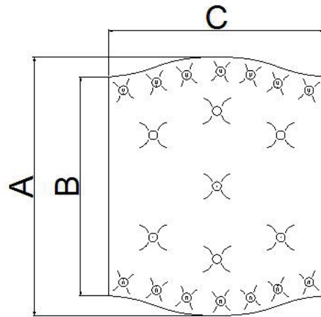
Fig. 1 - Dimensioni delle coibentazioni mod. IJ-FIG.
