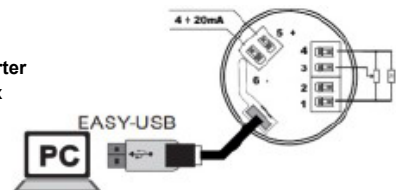
Converter a sicurezza intrinseca
