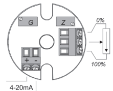
Converter a sicurezza intrinseca
