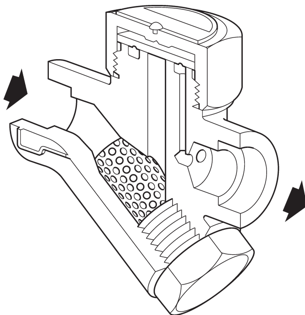
Fig. 1 - Scaricatore termodinamico TD42S2
