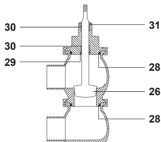
Fig. 5 - Valvola SH
