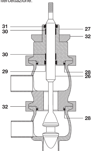
Fig. 2 - Valvola SQ
