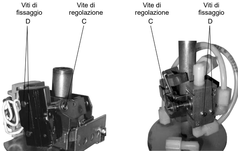
Fig. 7 - Interruttori elettrico e pneumatico
