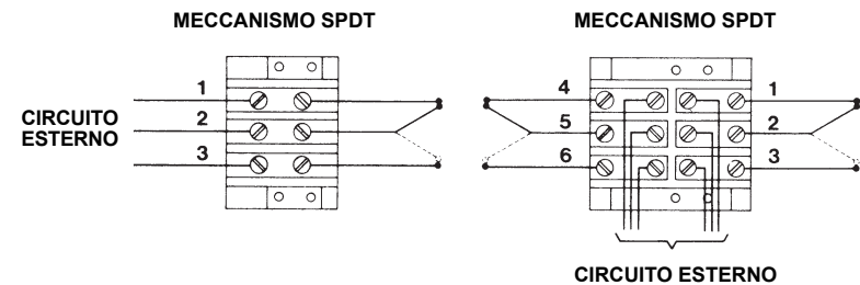
Fig. 3 - Schema elettrico dei meccanismi interruttori
