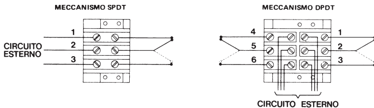
Fig. 3 - Schema elettrico dei meccanismi interruttori
