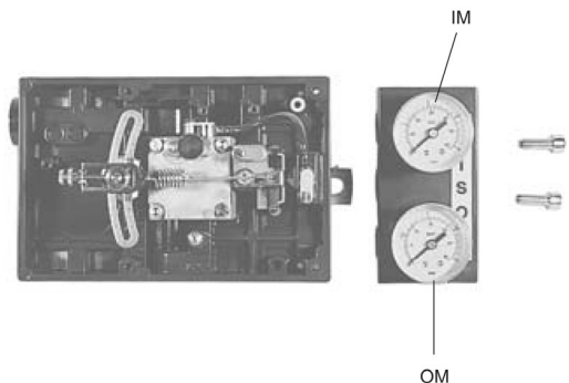
Fig. 13 - Gruppo manometri Gauges set
