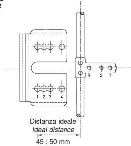
Fig. 5 - Selezione della corsa Stroke selection
