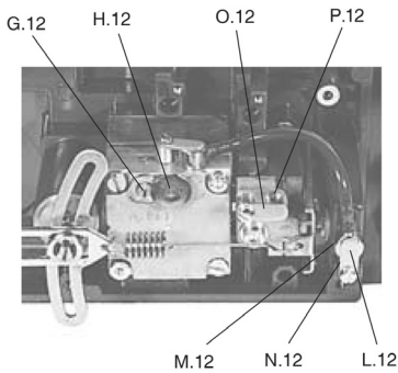
Fig. 12 - Gruppo ugelli Nozzle set
