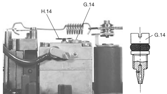
Fig. 14 - Gruppo orificio regolabile Adjustable orifice set
