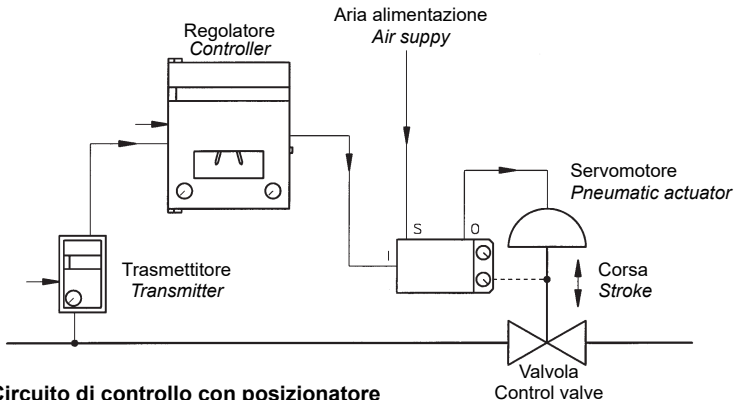
Fig. 1 - Circuito di controllo con posizionatore Control loop with positioner
