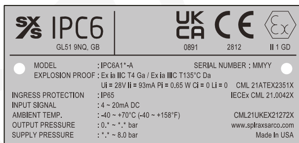
Fig. 1b Nameplate - UKEX / ATEX / IECEx
