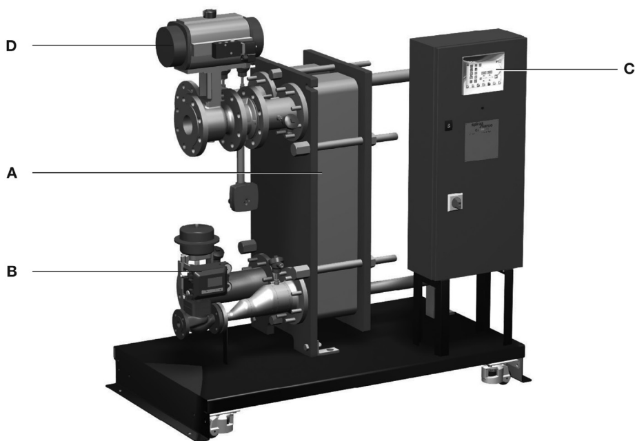
Fig. 1 - Unità compatta di scambio termico Spirax EasiHeat™ HTG
