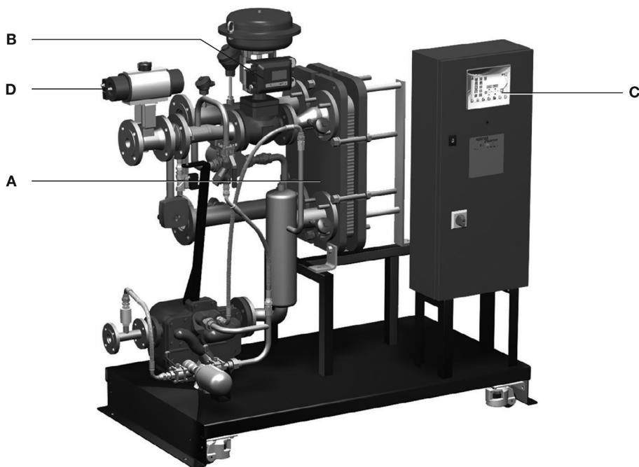
Fig. 1 - Unità di scambio termico Spirax EasiHeat™ DHW
