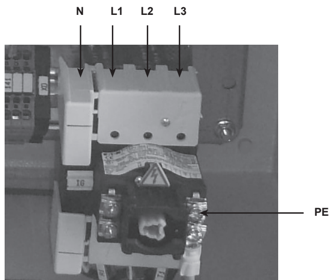
Fig. 7 Versione con alimentazione trifase + N
