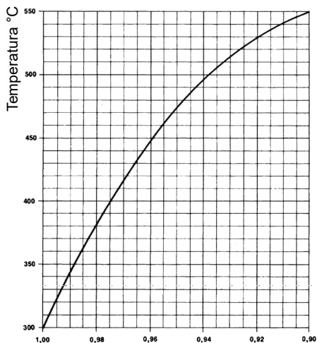
Coefficiente di riduzione del movimento e della pressione di esercizio in funzione della temperatura
