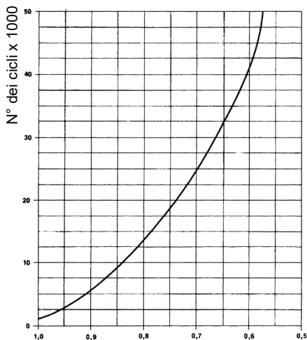
Coefficiente di riduzione del movimento in funzione dei cicli
