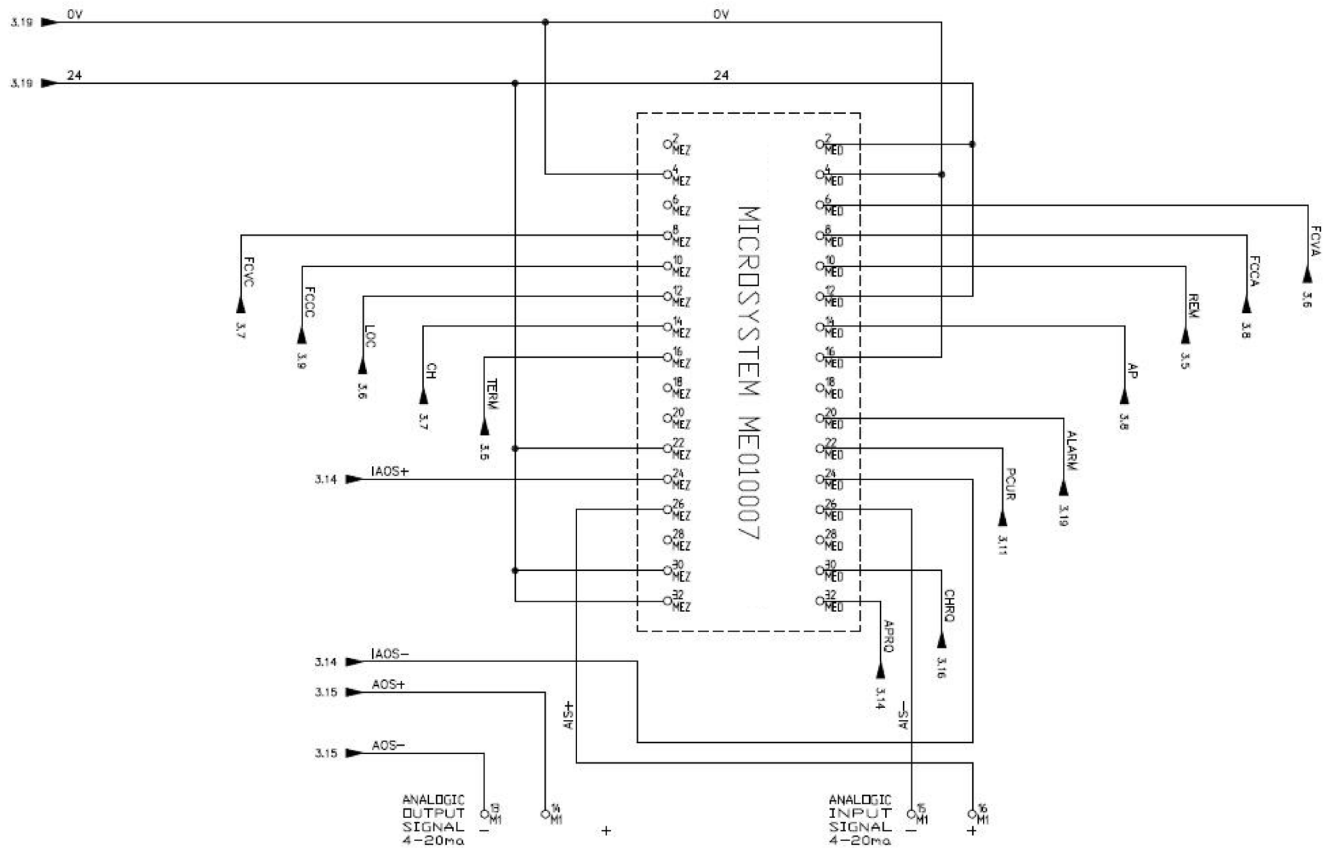
Fig. 12 - MDU100 Schemi elettrici
