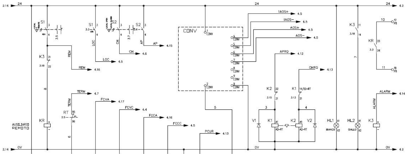
Fig. 11 - MDU100 Schemi elettrici
