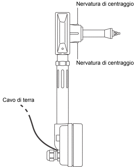
Fig. 15 - Nervature di centraggio incorporate
