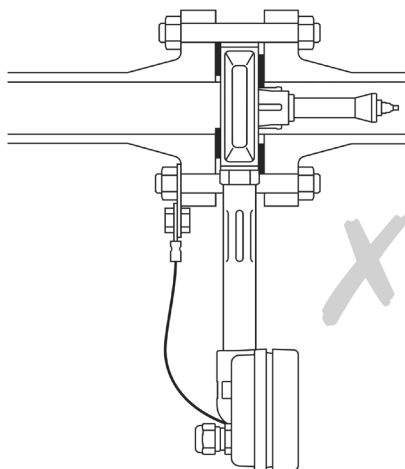
Fig. 17 - Guarnizione rientrante nella tubazione: montaggio non corretto
