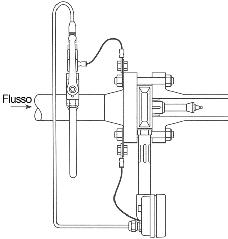
Fig. 9 - Flusso orizzontale fino a 32 bar per applicazioni su vapor saturo e fino a 23 bar g per applicazioni su vapore surriscaldato.
