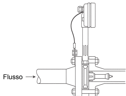
Fig. 8 - Flusso orizzontale limitato a 7 bar e alle sole applicazioni su vapore saturo
