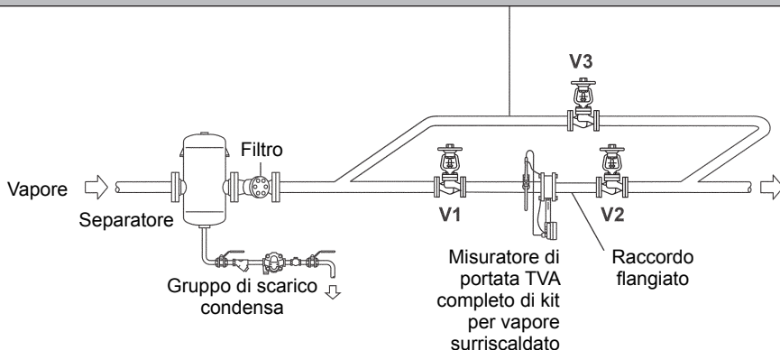
Fig. 5 - Installazione tipica
