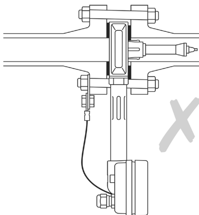
Fig. 18 - Guarnizione e tubazioni disassate: montaggio non corretto
