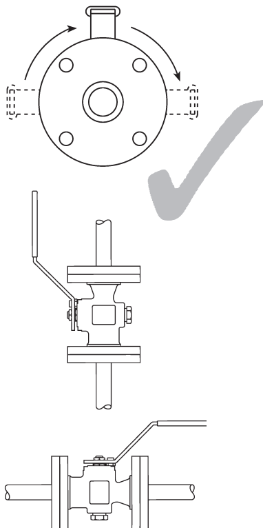
Fig. 3 - Installazione corretta per impieghi con i gas
