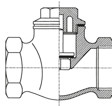
Fig. 6 Valvola di ritegno RJ205N
