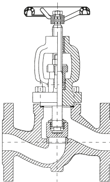
Fig. 2 Valvola di intercettazione GXM16Z
