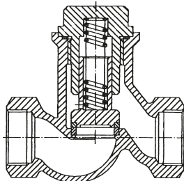
Fig. 5 Valvola di ritegno RJ205Z
