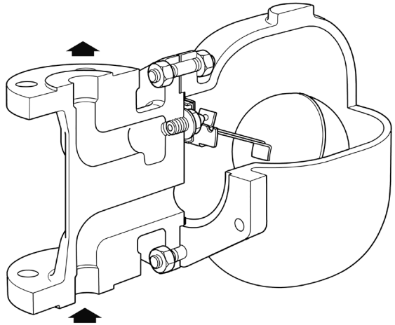
Fig. 4 - AE44S DN25
