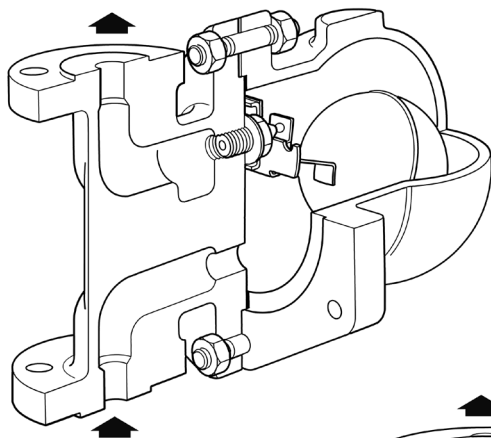
Fig. 1 - AE44 DN15 e DN20
