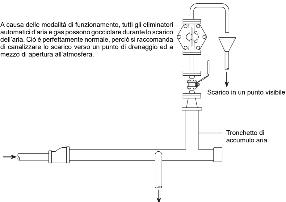
Fig. 6 - Applicazione tipica che mostra un eliminatore d'aria AE44 installato su impianto idronico ad alta temperatura (HTHW).
