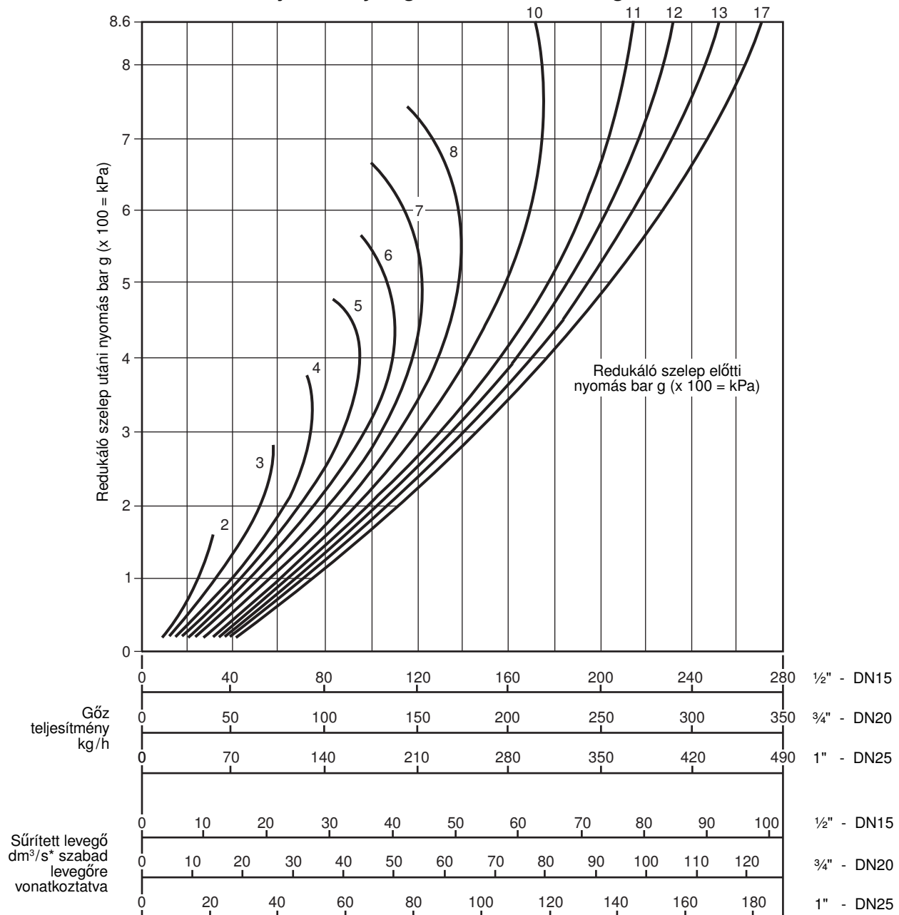
Teljesítmények gőzre és sűrített levegőre
