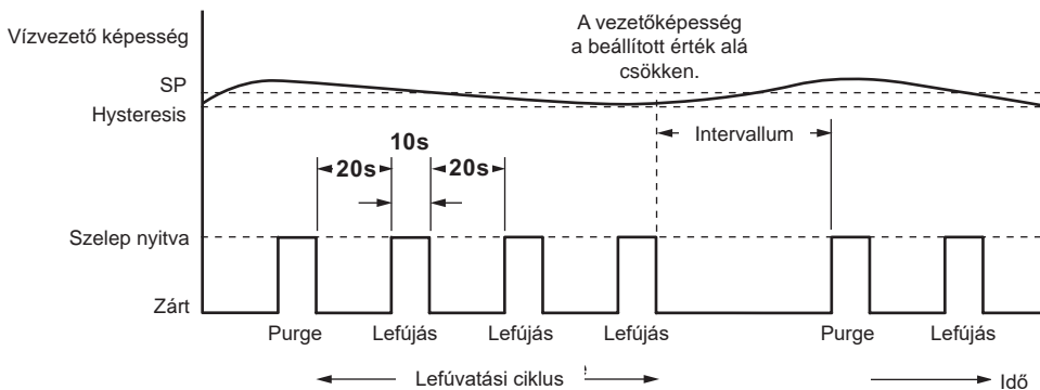
18. ábra: BE/KI vezérlés átfúvatással és impulzuskimenettel
