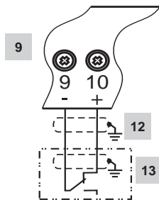
7. ábra Alsó iszapoló kapcsoló csatlakozás (az ábrán a szelep zárva)
