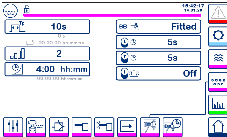
40. ábra: Alsó iszapolás korlátozó kapcsolójának paraméterei
