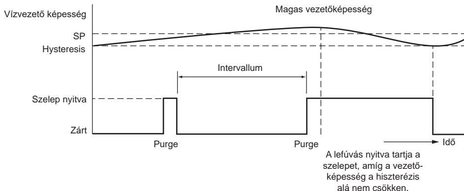
17. ábra: BE/KI vezérlés átfúvatással
