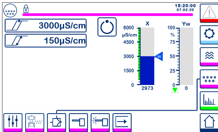
31. ábra: BE/KI vezérlési paraméterek
