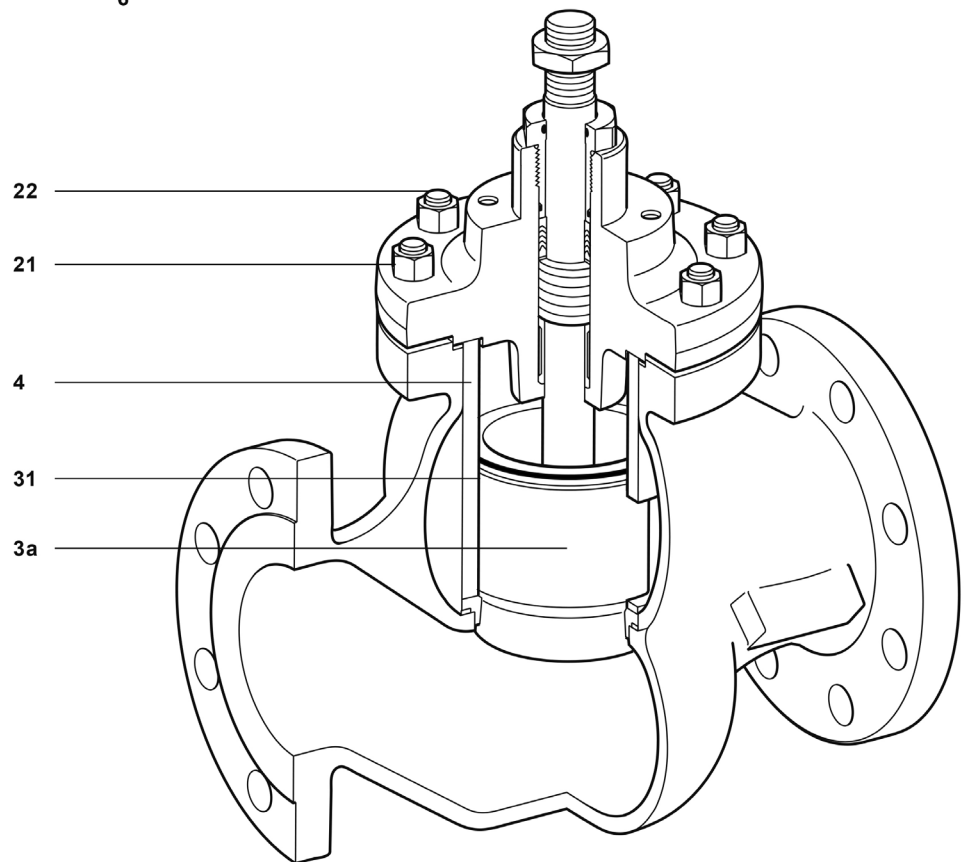
Vanne équilibrée DN125
