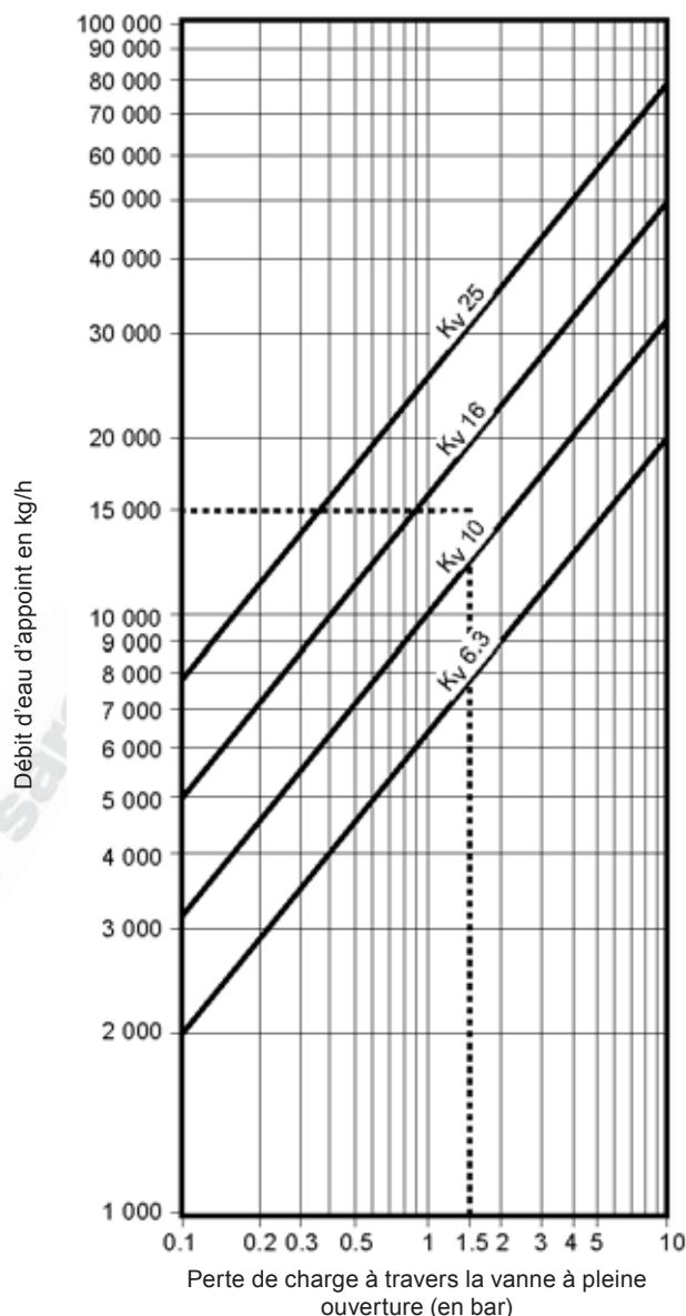
Diagramme de sélection du Kv de la vanne
