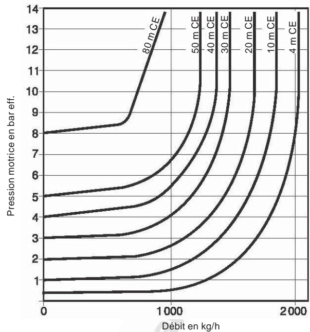
Débits de la pompe en DN40
