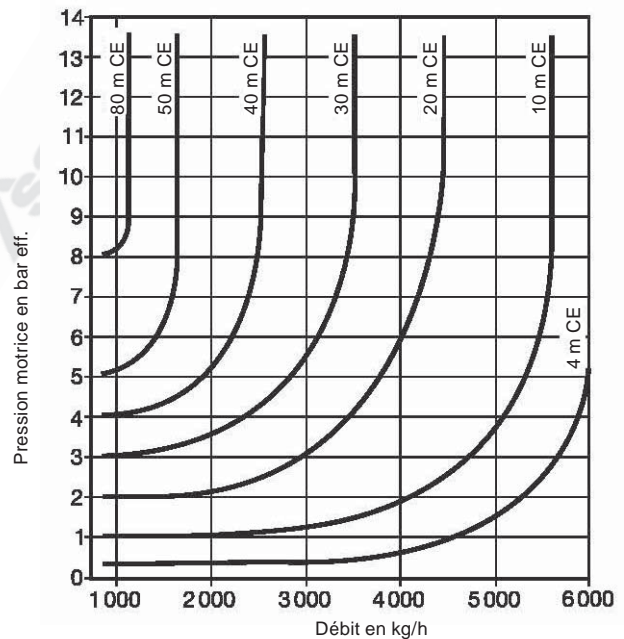
Débits de la pompe en DN80 x DN50
