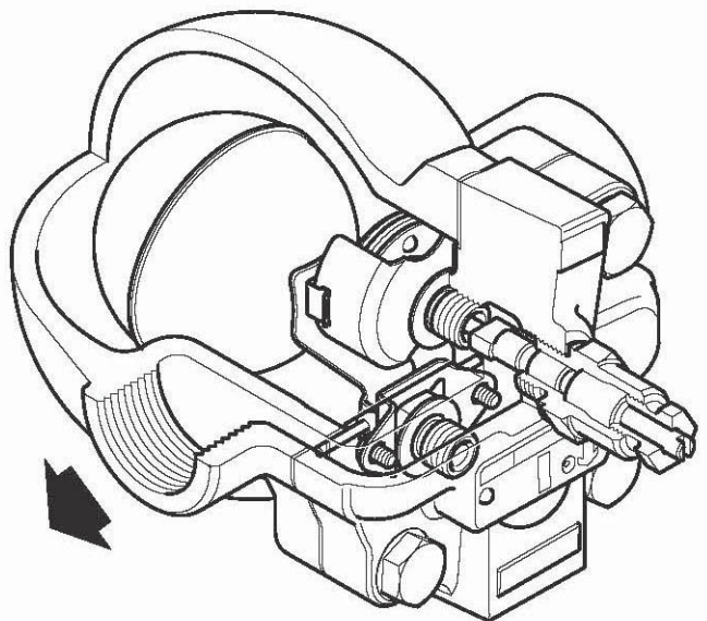
FTGS14-C (R-L) (avec système anti-bouchon de vapeur (SLR) en option)
