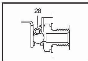
Ensemble clapet principal pour 1"
