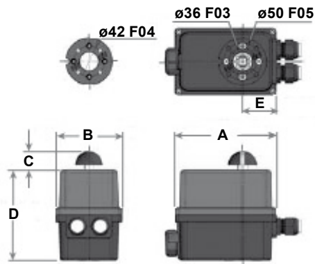
BVE ER 35 - ER60 - ER 100
